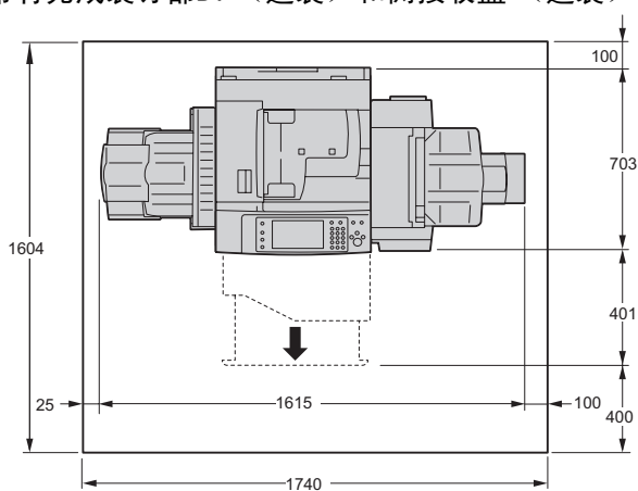
带有完成装订部B1（选装）和侧接收盘（选装）
