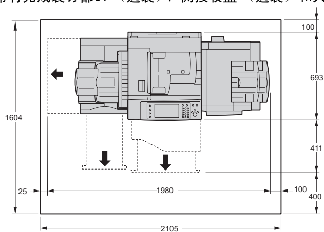
带有完成装订部C1（选装）、侧接收盘（选装）和大容量纸盘（选装）
