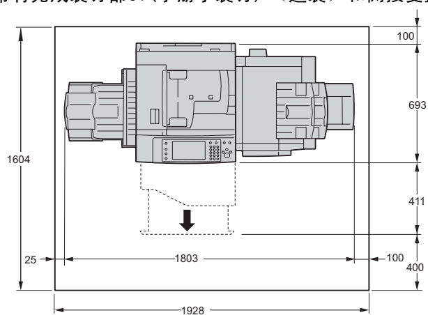
带有完成装订部C1（小册子装订）（选装）和侧接受盘（选装）
