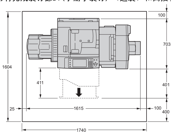
带有完成装订部B1（小册子装订）（选装）和侧接收盘（选装）
