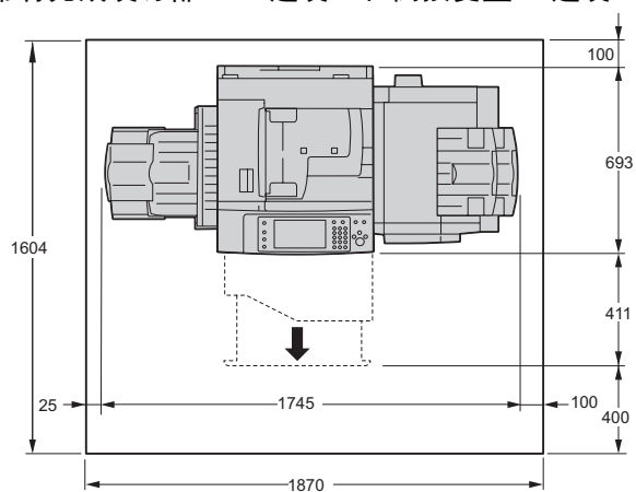
带有完成装订部C1（选装）和侧接受盘（选装）
