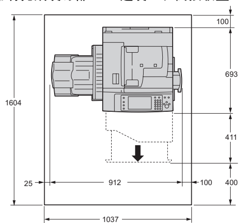
带有完成装订部A1（选装）和侧接收盘（选装）
